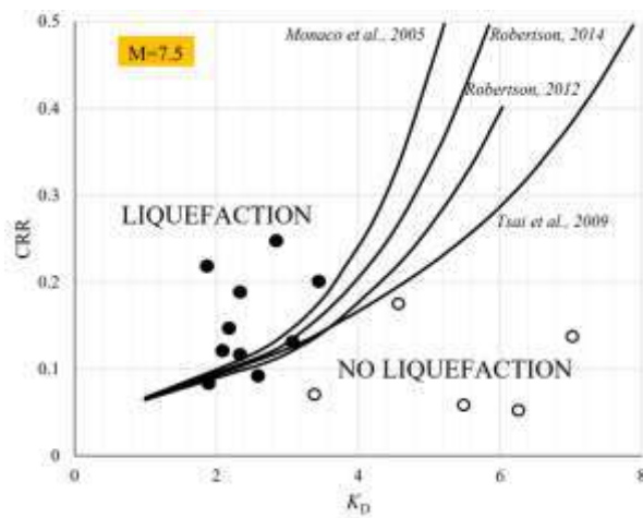
FIG. 6(C) DMT
