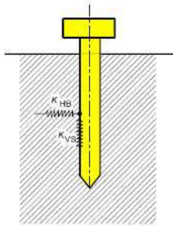
FIG. 3B PILE
