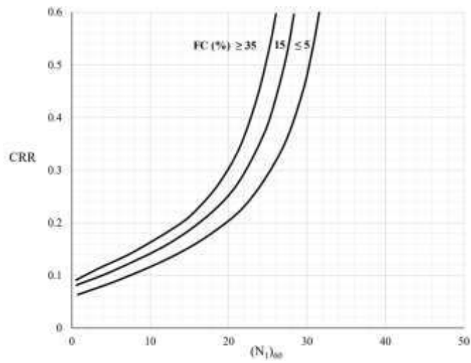
FIG. 6(B) SPT
